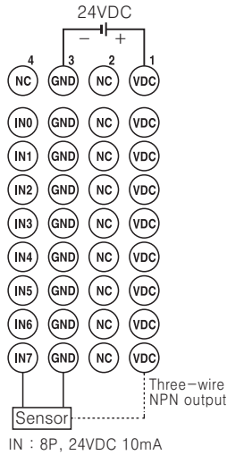
ARD-DI08N-4S
